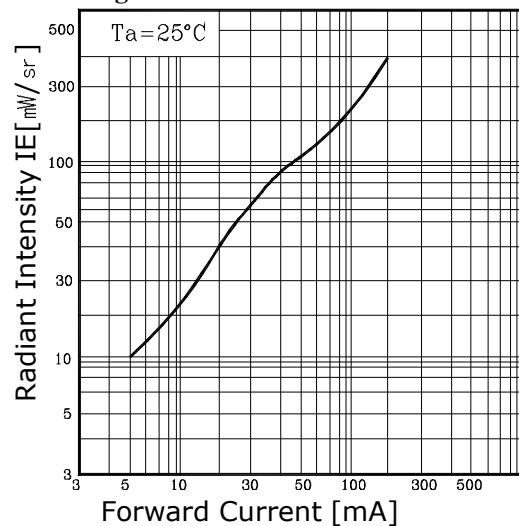
Fig.4 I_e - I_F
