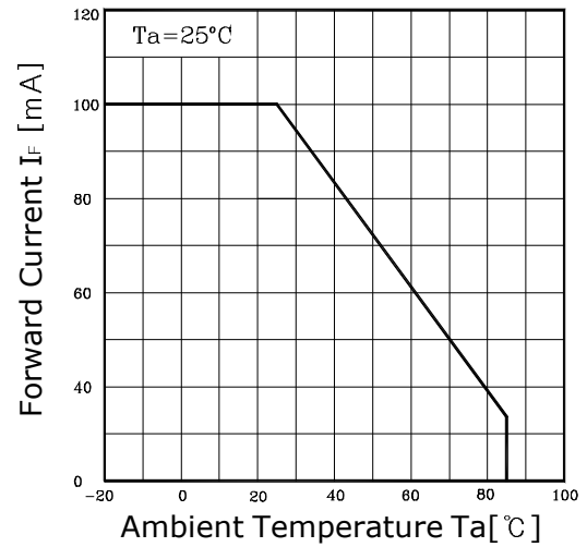
Fig.2 I_F - T_a
