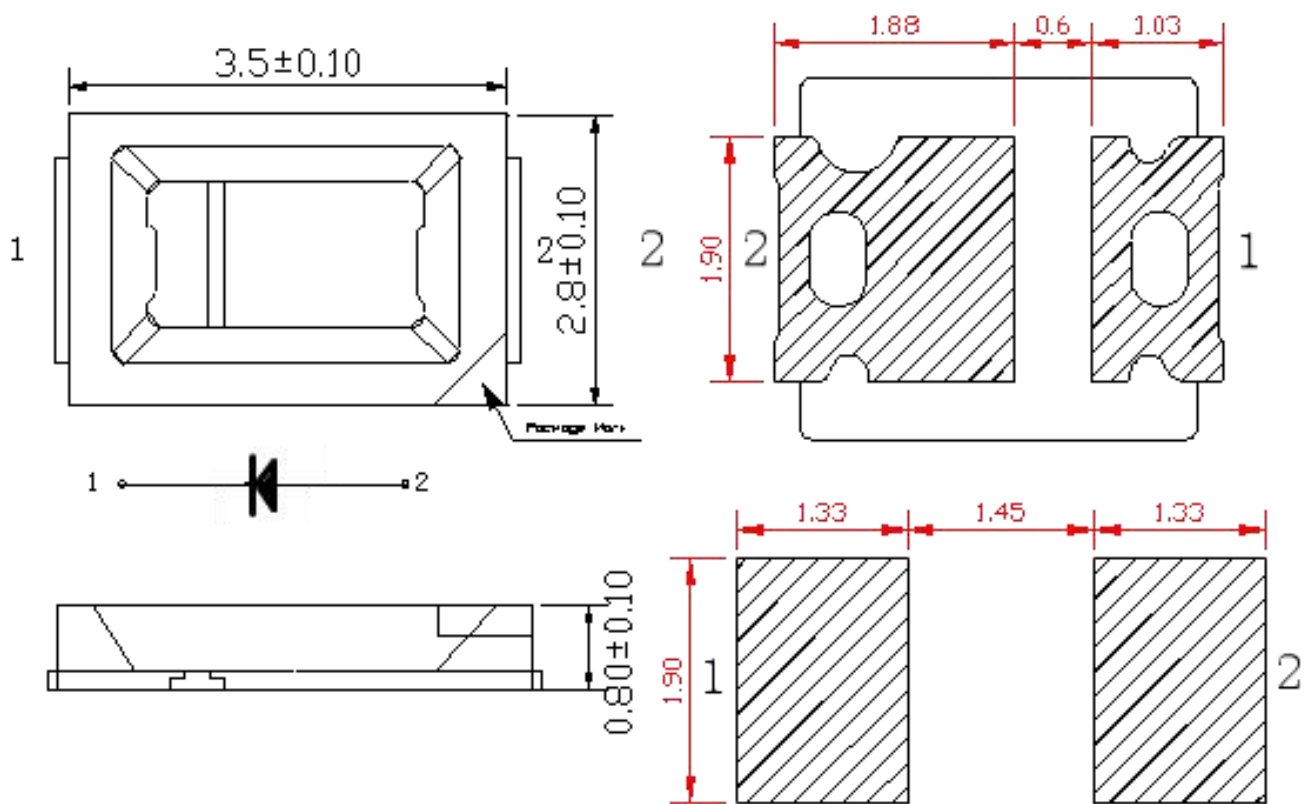
焊盘图
