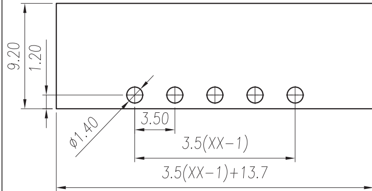
P.C.B. LAYOUT
