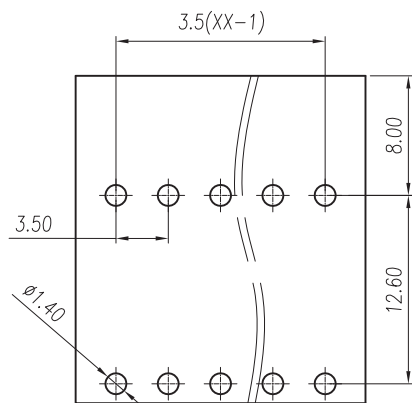
P.C.B. LAYOUT
