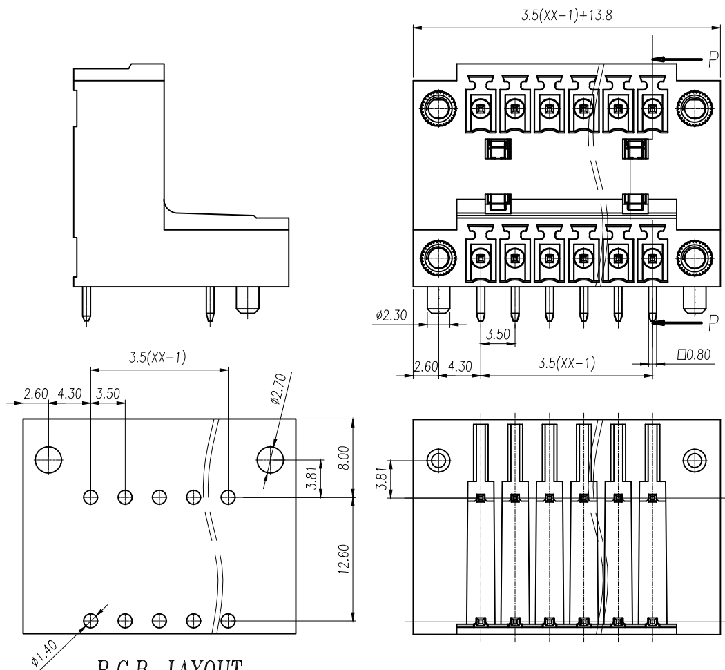
P.C.B. LAYOUT
