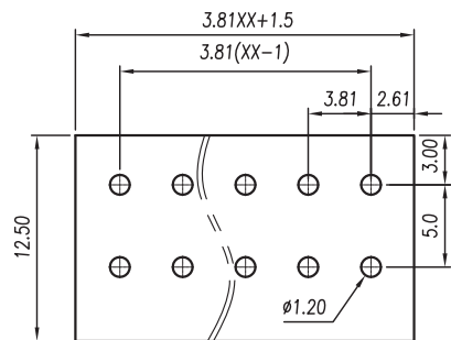
P.C.B. LAYOUT
