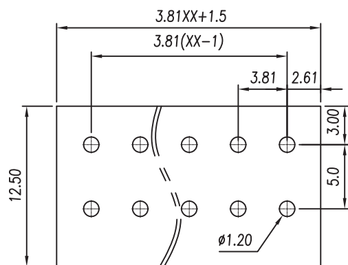
P.C.B. LAYOUT
