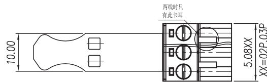
02~03P尺寸图
