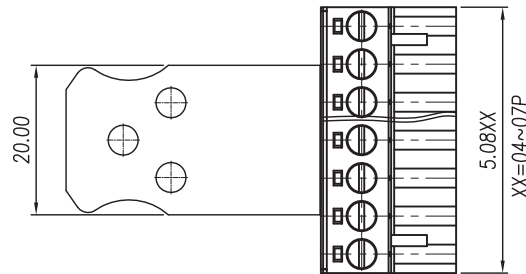
04~07P尺寸图
