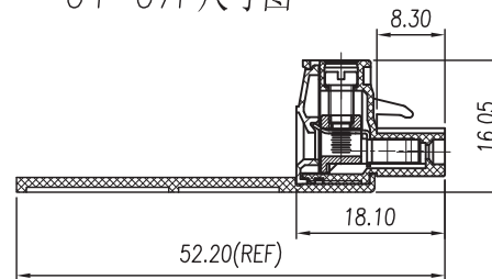
04~07P尺寸图
