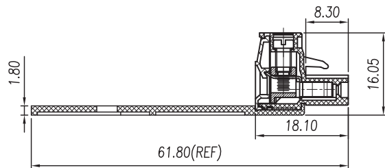
08~24P尺寸图
