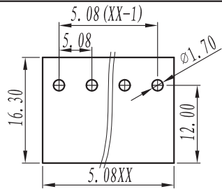
P.C.B. LAYOUT S=1:2
