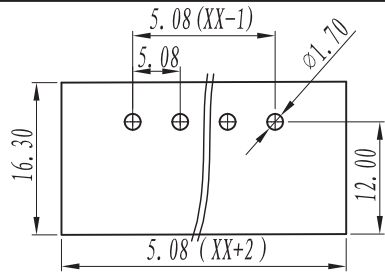
P.C.B. LAYOUT S=1:2
