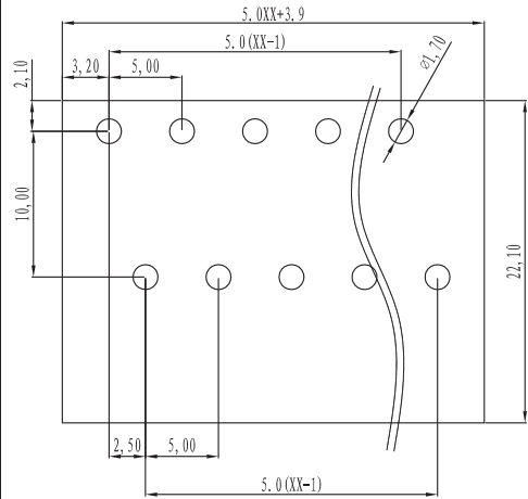
P.C.B. LAYOUT
