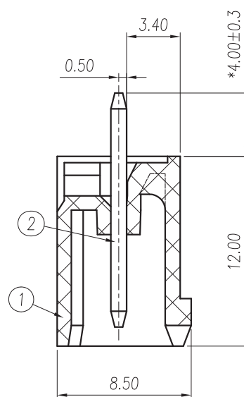
SECTION:A-A
