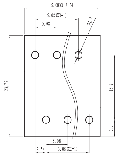
P.C.B. LAYOUT
