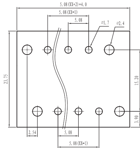
P.C.B. LAYOUT
